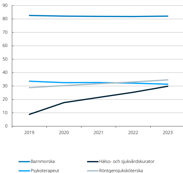
Figur 1. Total antal utfärdade legitimationer, under 65 år
